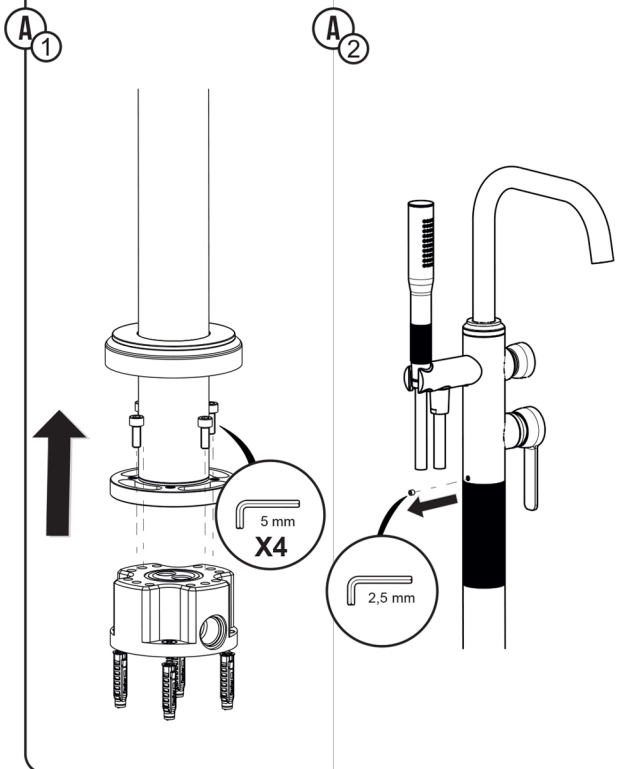
Cambio flessibile | Flexible hoses replacement | Sustitución de los latiguillos de alimentación | Flexible Schaltgetriebe | Sustitución de los latiguillos de alimentación
