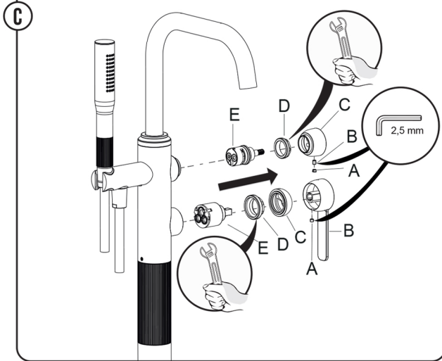
Cambio cartuccia | Cartridge change | Changement de cartouche | Austausch Kartusche | Cambio de cartucho
