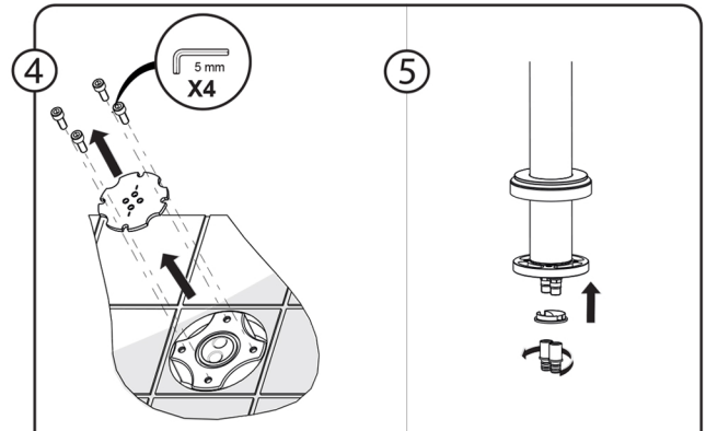
Cambio cartuccia | Cartridge change | Changement de cartouche | Austausch Kartusche | Cambio de cartucho
