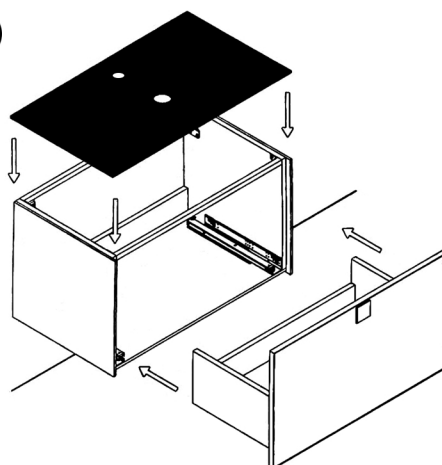
installazione del piano ed inserimento del cassetto su guida Top board fixing on frame and drawer onto rails
