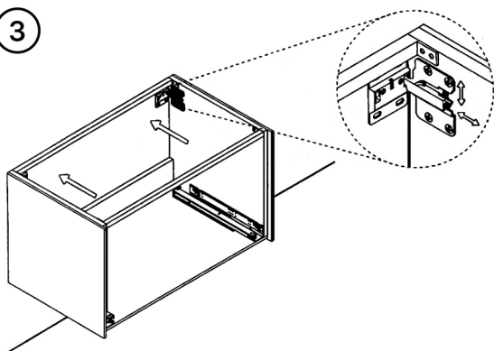
Ancoraggio e registrazione della consolle Unit anchoring and adjustment
